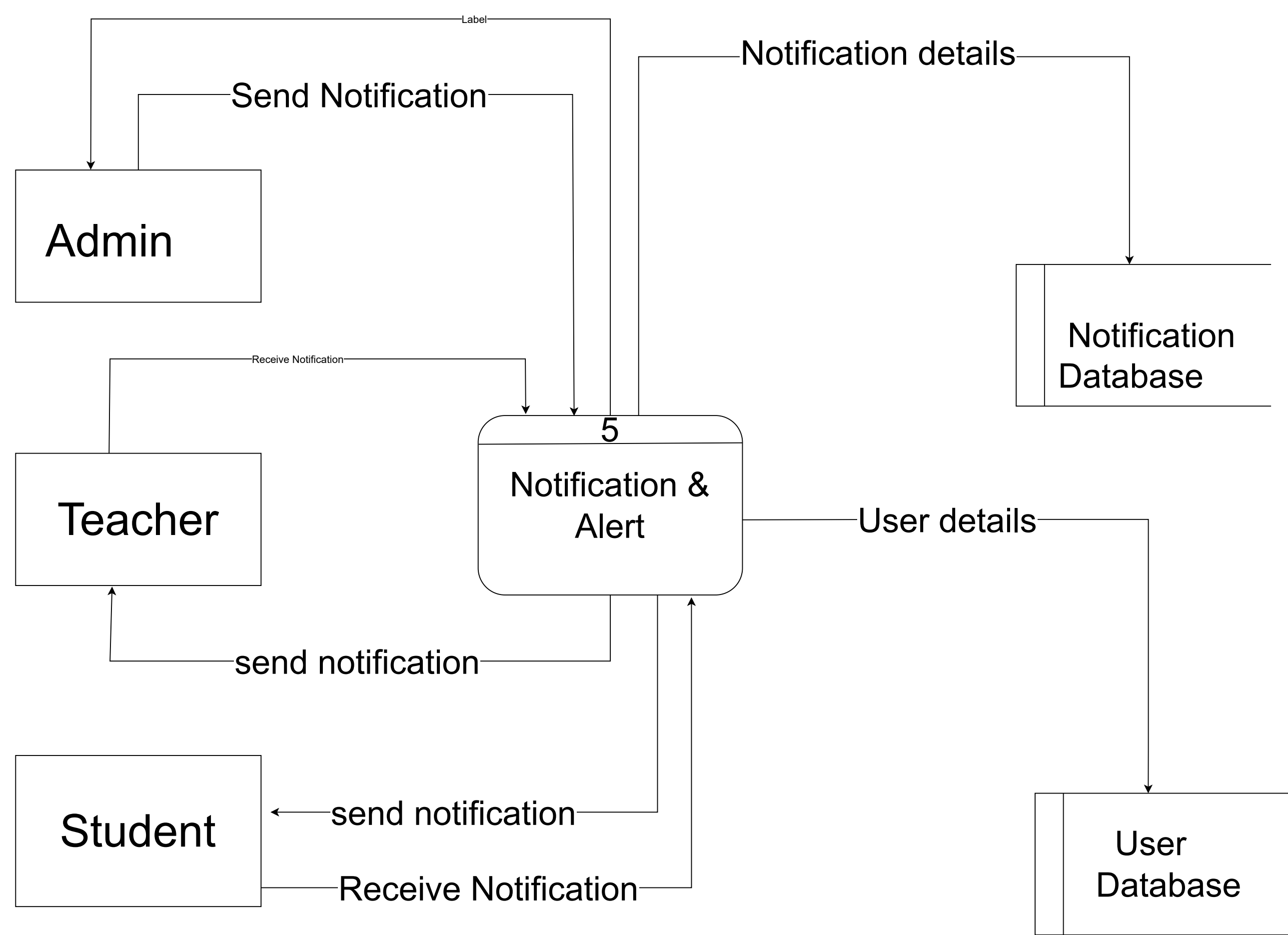
DFD Level 2
