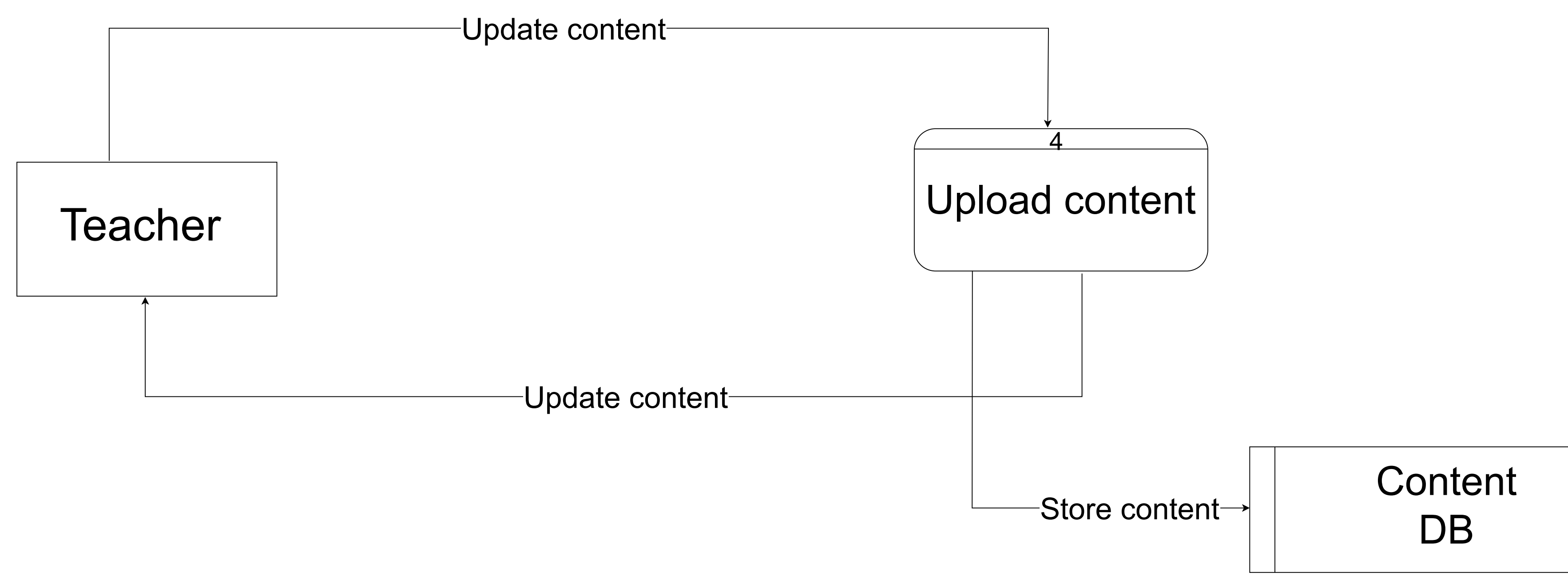
DFD Level 2
