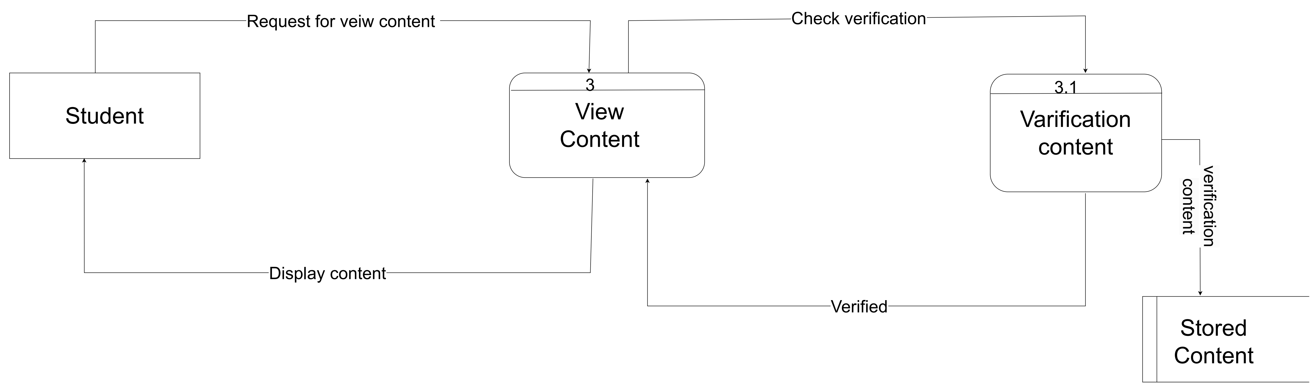
DFD Level 2
