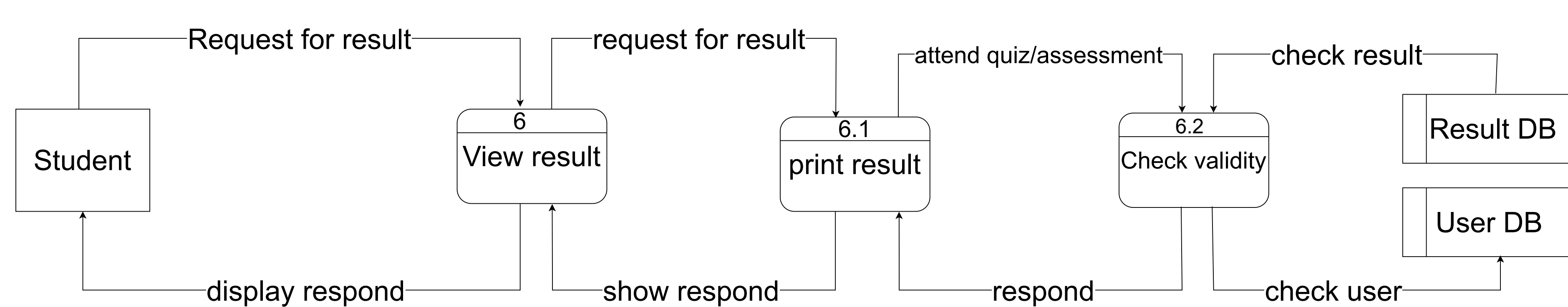
DFD Level 2
